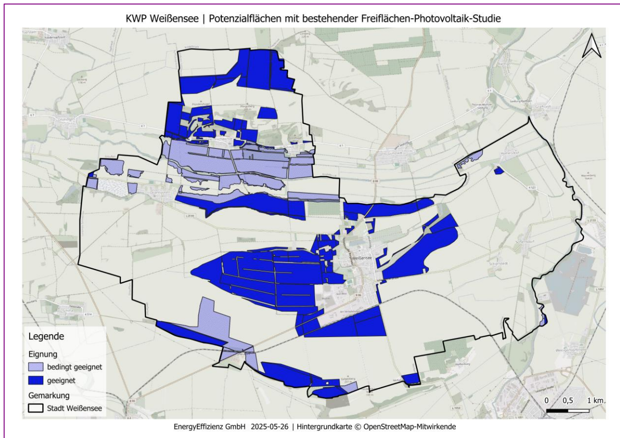
Abbildung 23: Potenzialflächen Freiflächen-Photovoltaik
