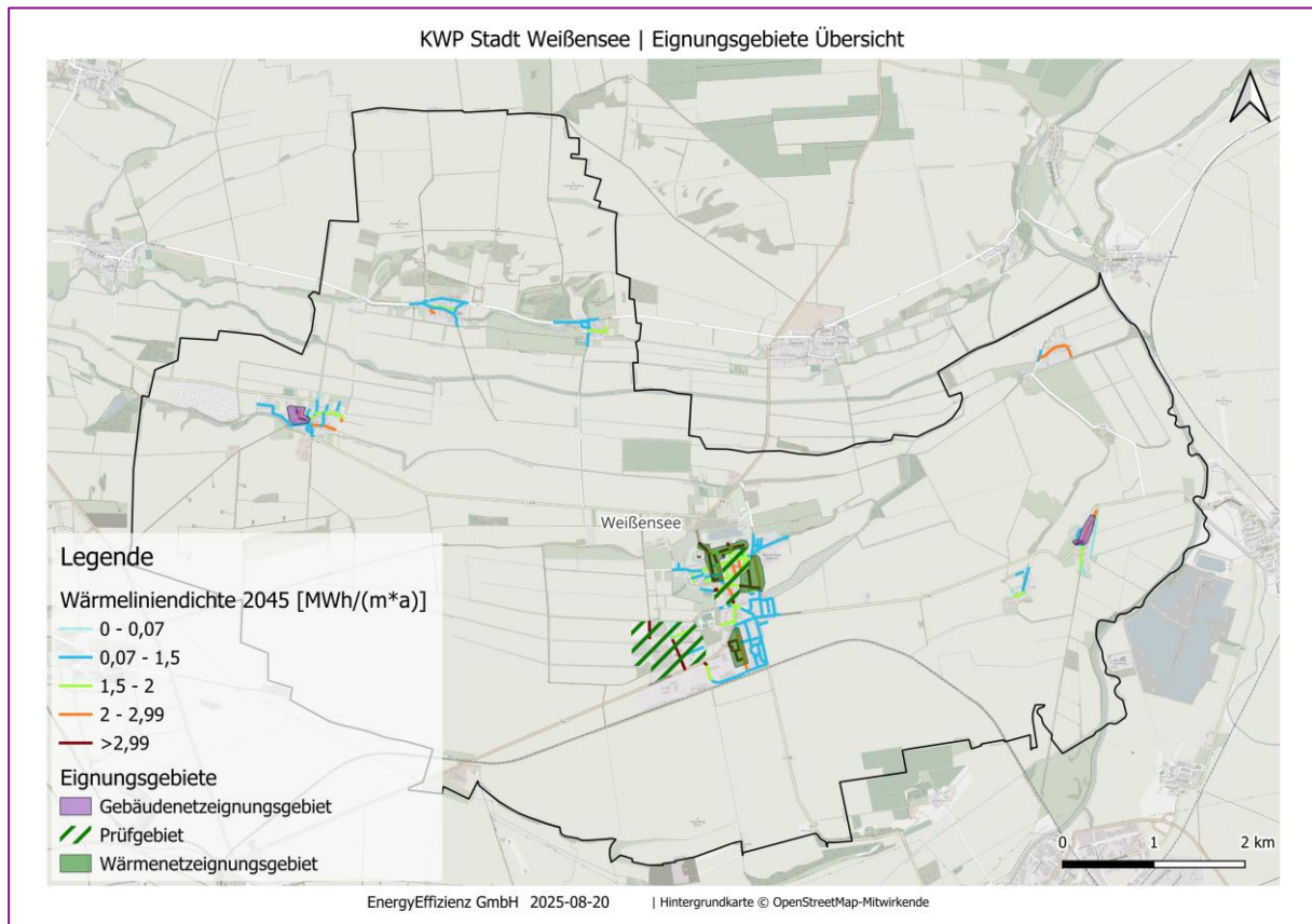
Abbildung 26: Eignungsgebiete in der Stadt Weißensee (Thüringen) inkl. Ortsteile
