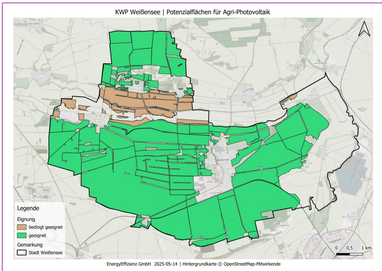
Abbildung 24 Potenzialflächen Agri-PV
