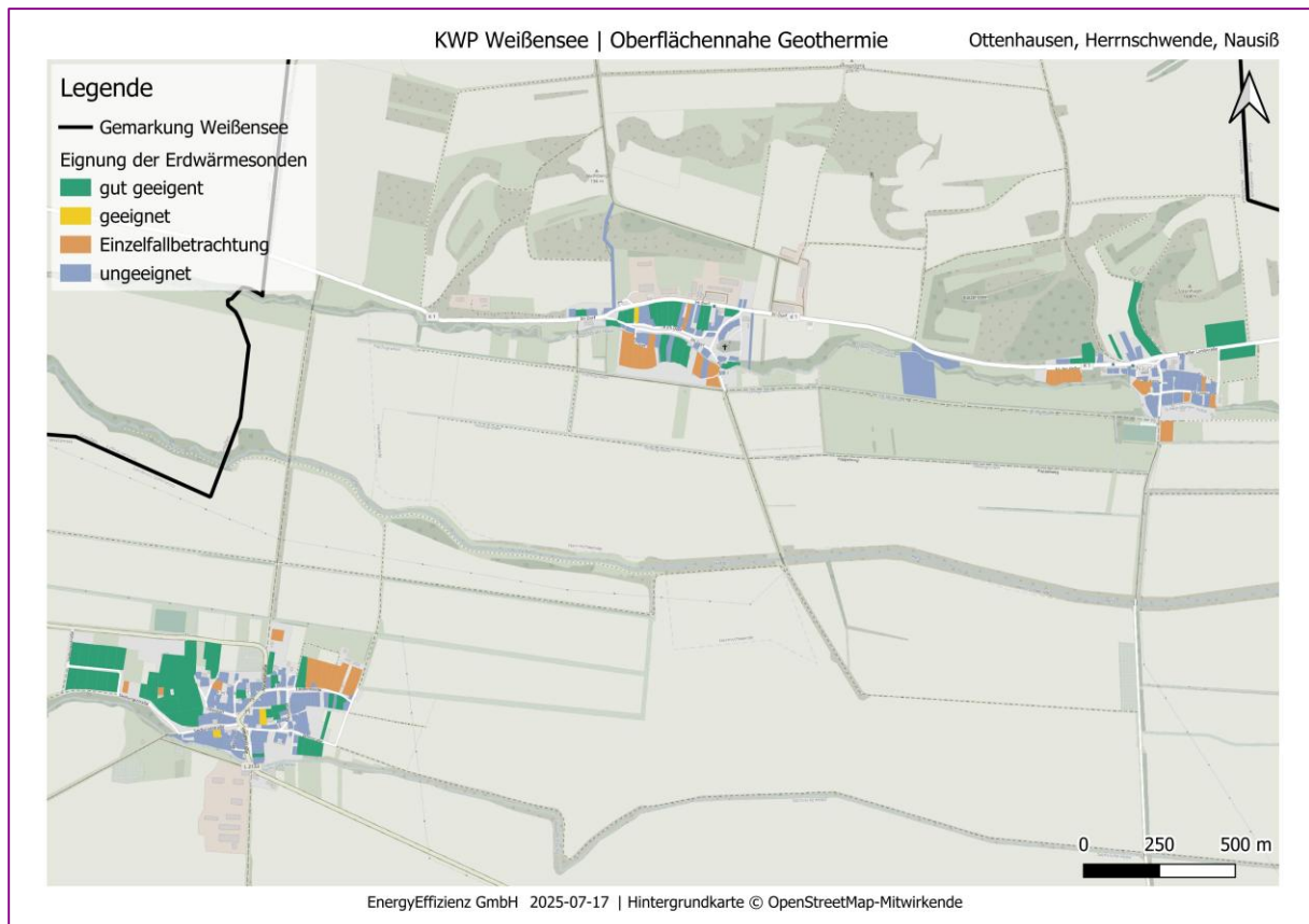
Abbildung 44: Eignung Erdwärmesonden in den Stadtteilen Ottenhausen, Herrnschwende und Nausiß
