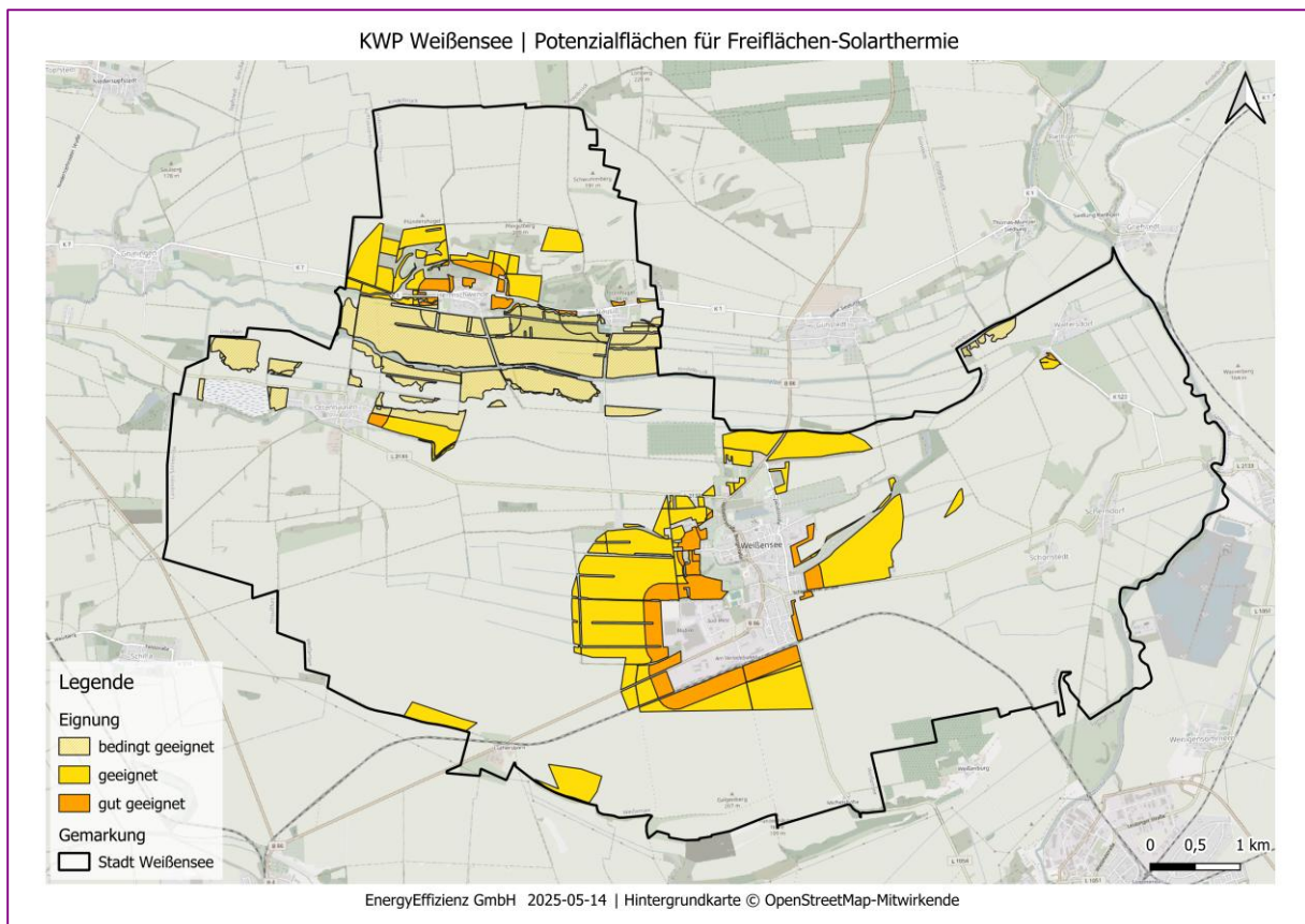
Abbildung 17: Potenzialflächen Freiflächen-Solarthermie
