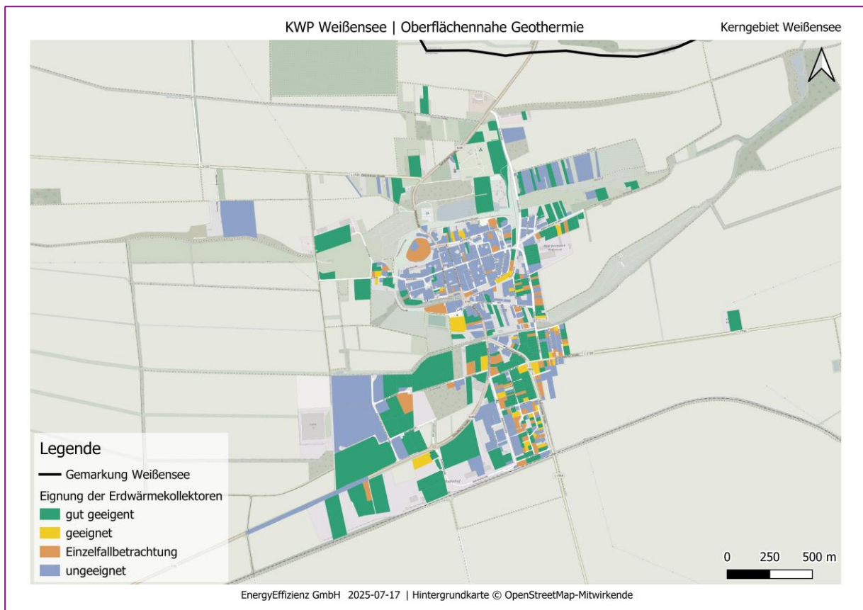
Abbildung 43: Eignung Erdwärmekollektoren in Weißensee (Thüringen)
