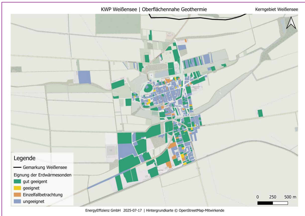
Abbildung 22: Eignung von Erdwärmesonden auf Flurstücksebene in Weißensee (Thüringen)
