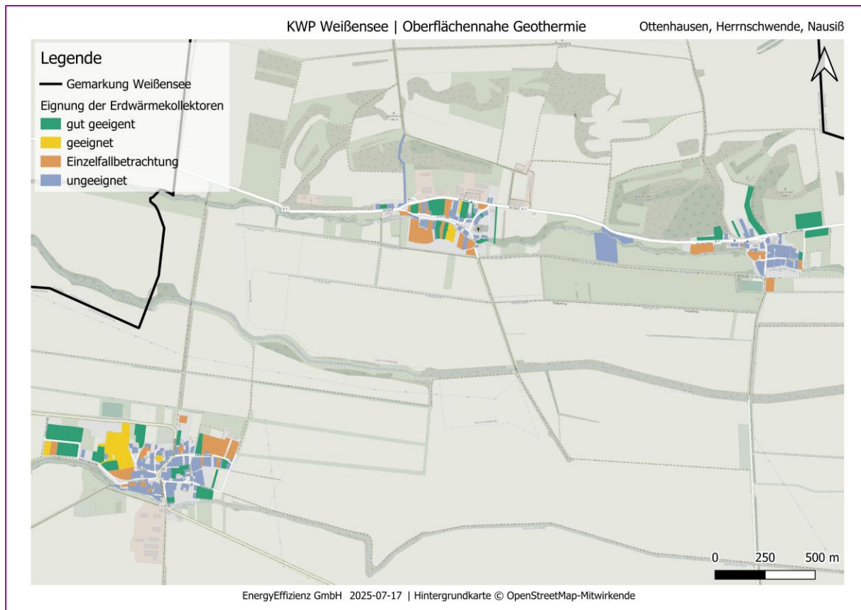
Abbildung 41: Eignung Erdwärmekollektoren in den Stadtteilen Ottenhausen, Herrnschwende und Nausiß
