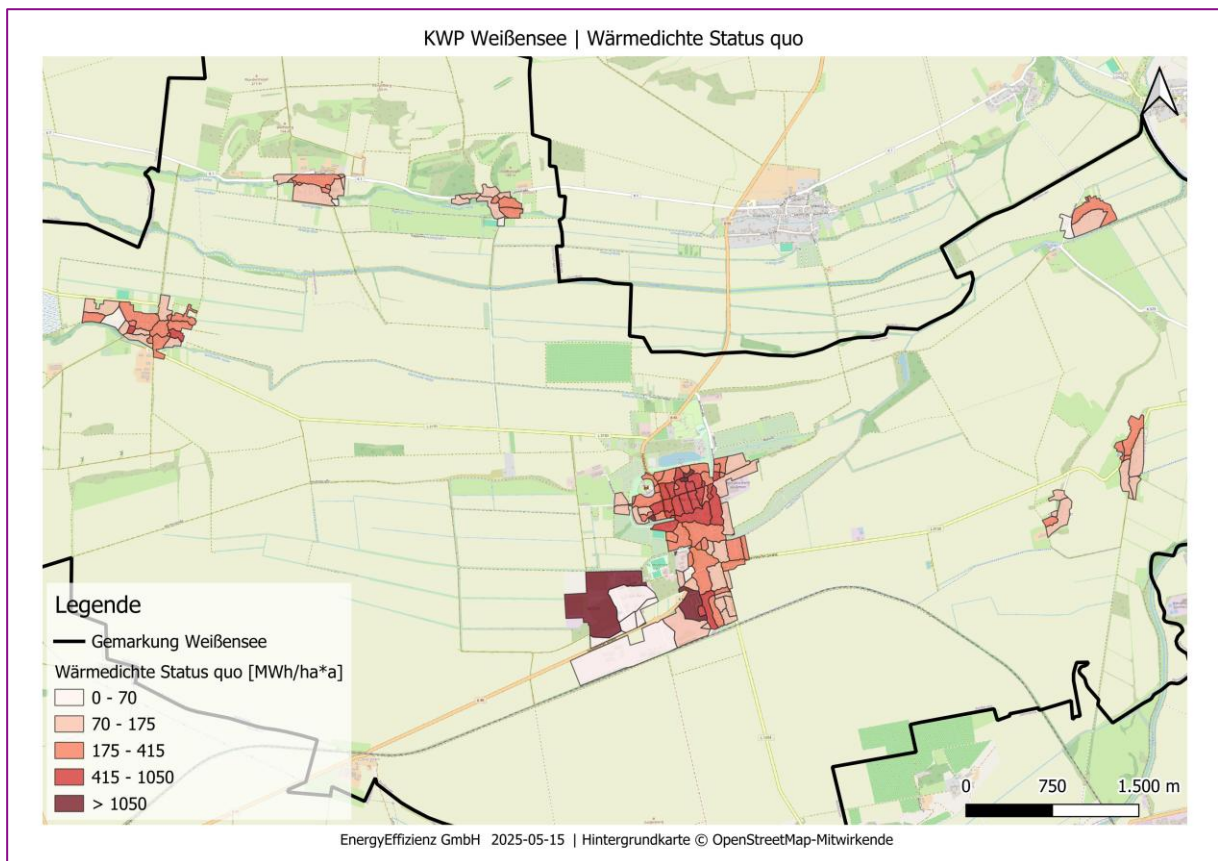
Abbildung 13: Wärmedichte je Baublock Status quo in Weißensee (Thüringen)
