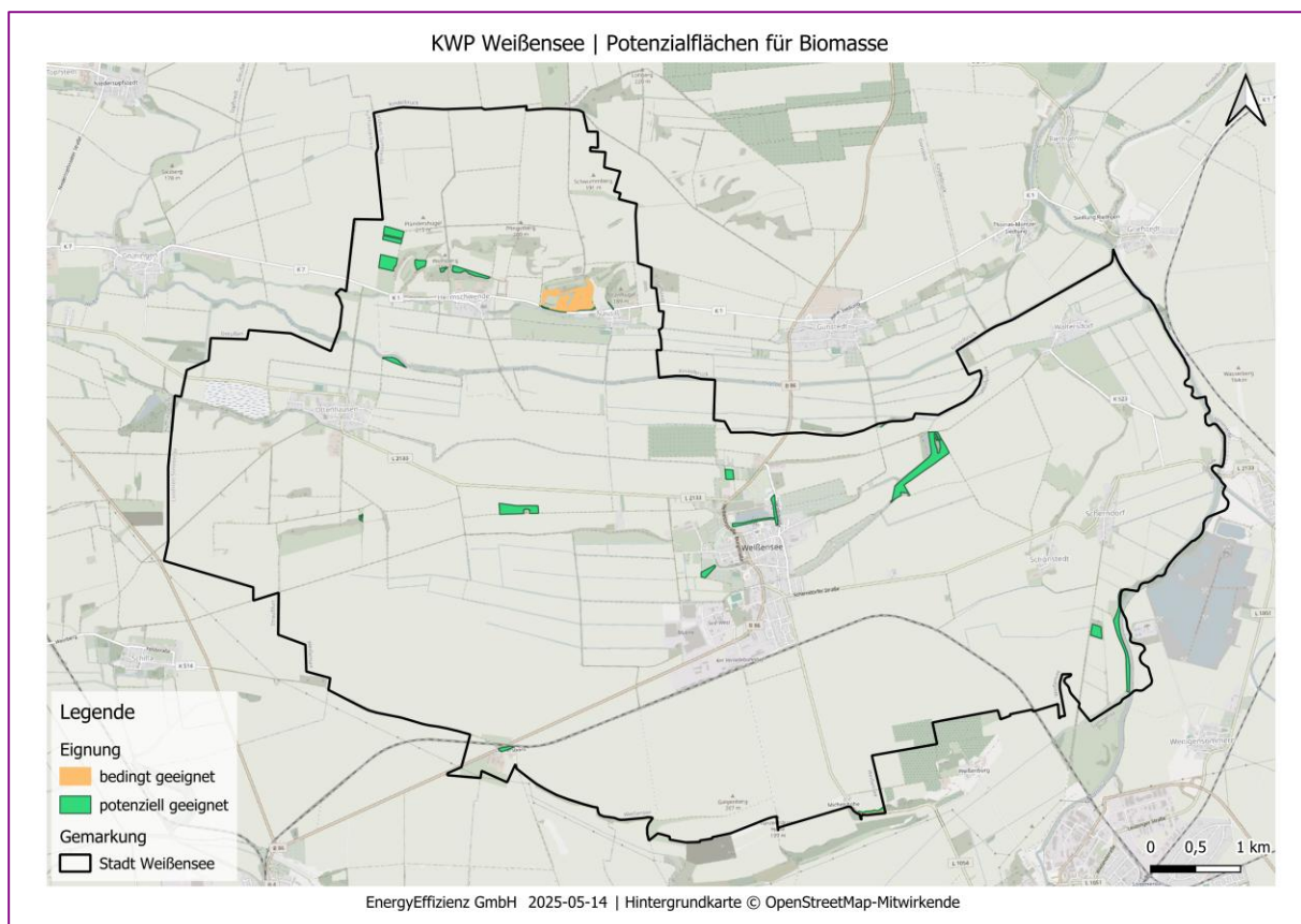
Abbildung 16: Biomassepotenzial in Weißensee
