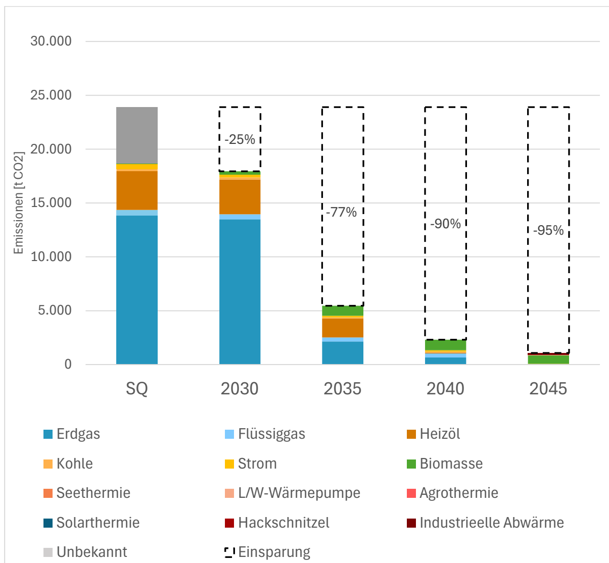
Abbildung 35: Emissionssenkung bis 2045 gemäß Zielszenario
