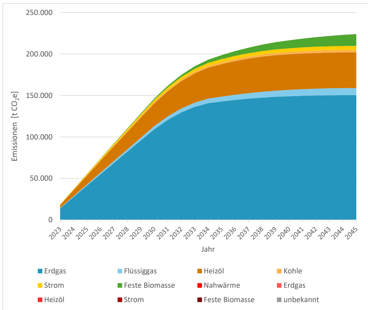
Abbildung 36: Kumulierte CO 2 -Emissionen bis 2045
