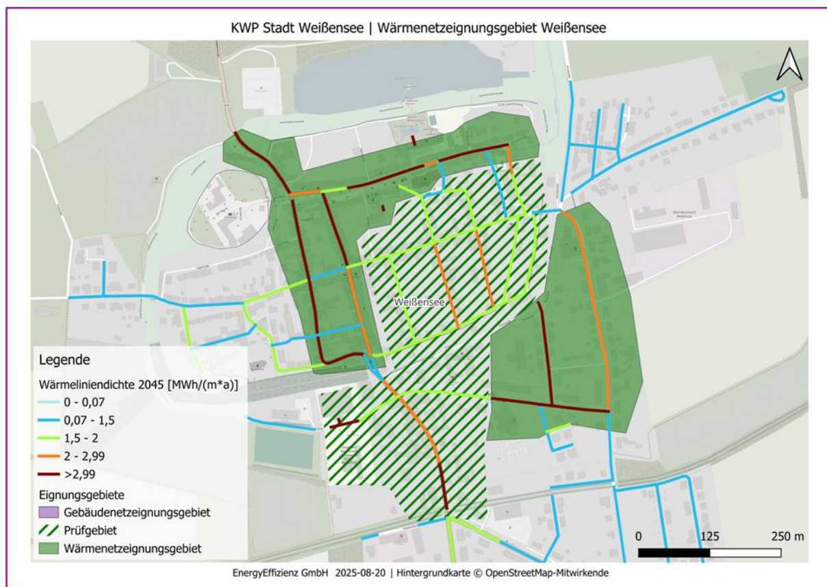
Abbildung 37: Fokusgebiet 1 – Wärmenetzeignungsgebiet in dem Zentrum von Weißensee
