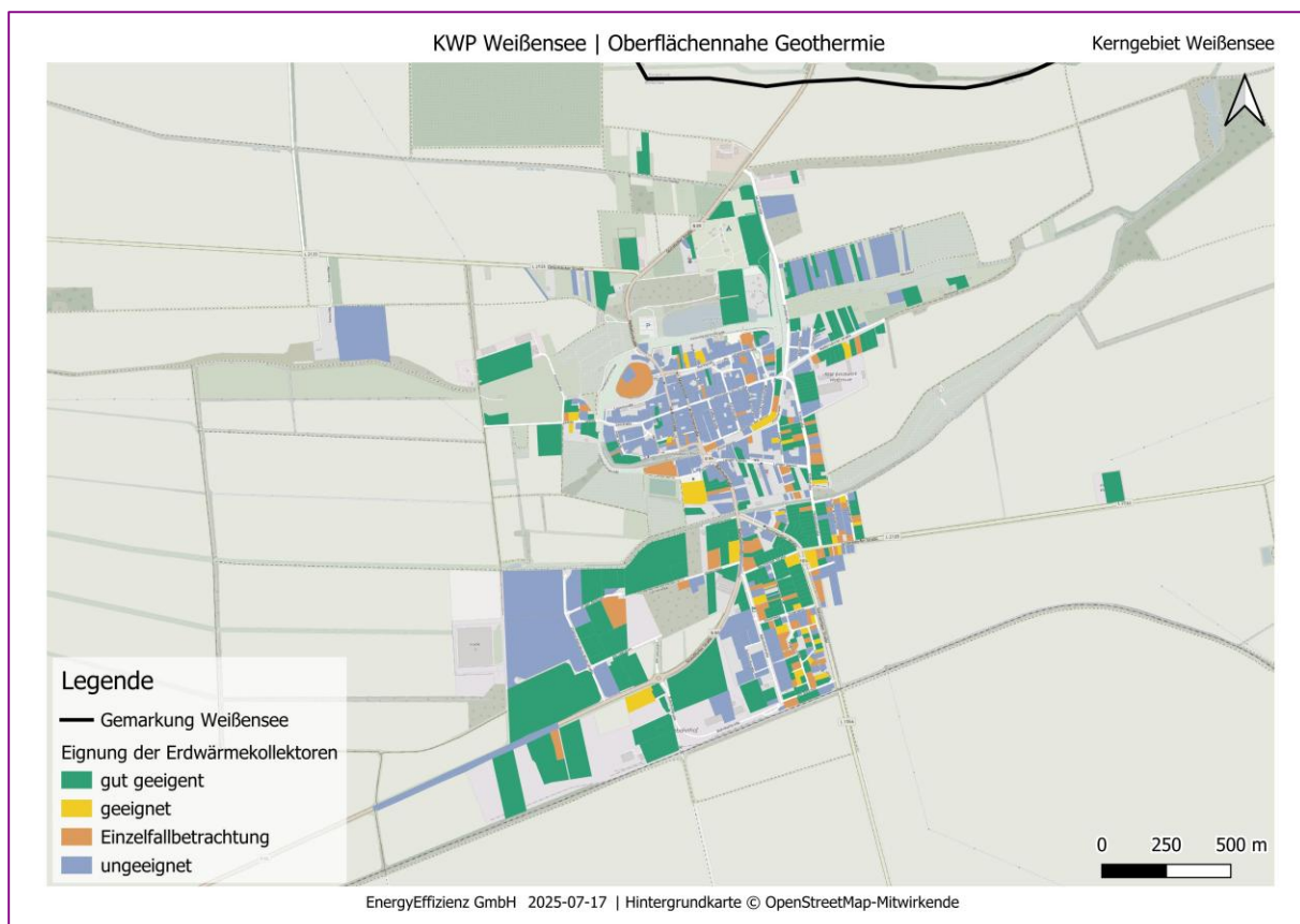
Abbildung 21: Eignung von Erdwärmekollektoren in Weißensee (Thüringen)
