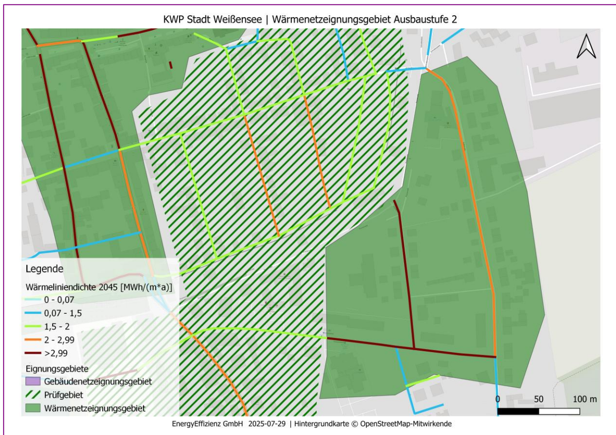
Abbildung 31: Wärmenetz Weißensee (Thüringen) Ortszentrum Ost, 100 % Anschlussquote
