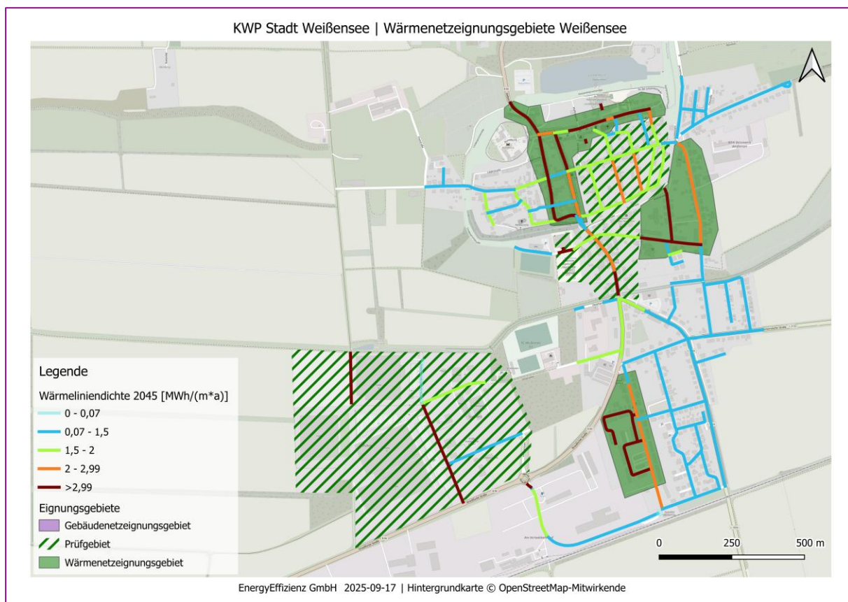
Abbildung 27: Eignungsgebiete in der Stadt Weißensee (Thüringen)
