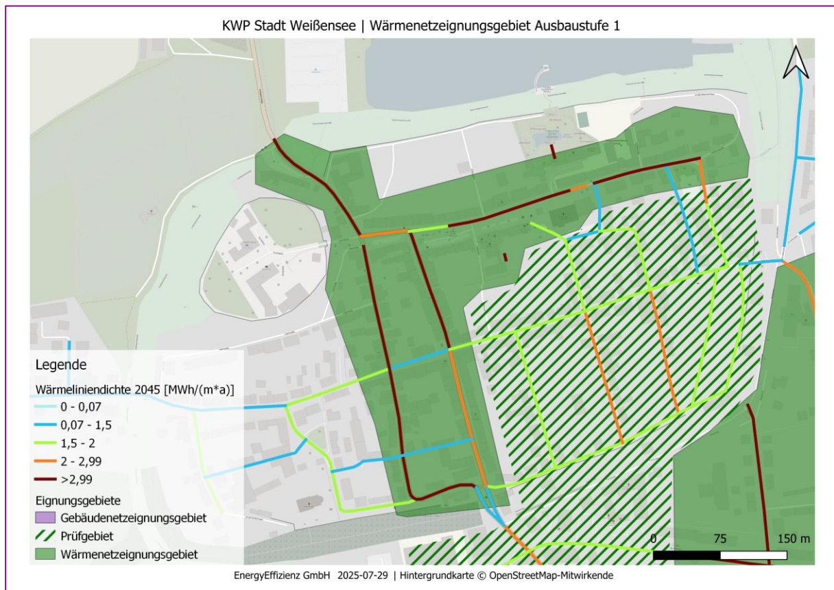
Abbildung 29: Wärmenetz Weißensee (Thüringen) Ortszentrum Nord, 100 % Anschlussquote
