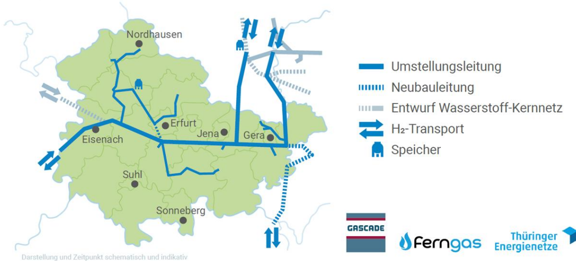
Abbildung 20: Geplantes Wasserstoffnetz in Thüringen 2032
